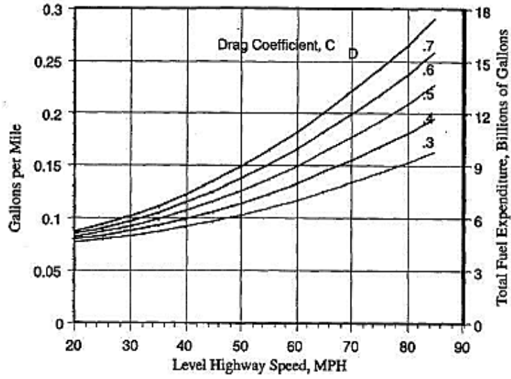
الشكل (١) يمثل زيادة صوفيات الوقود مع زيادة قوى الكبح [7].
