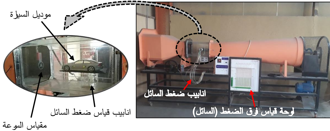
الشكل (٢) يبين النفق الهوائي و الموديل المستخدم لاجراء التجارب العملية.
