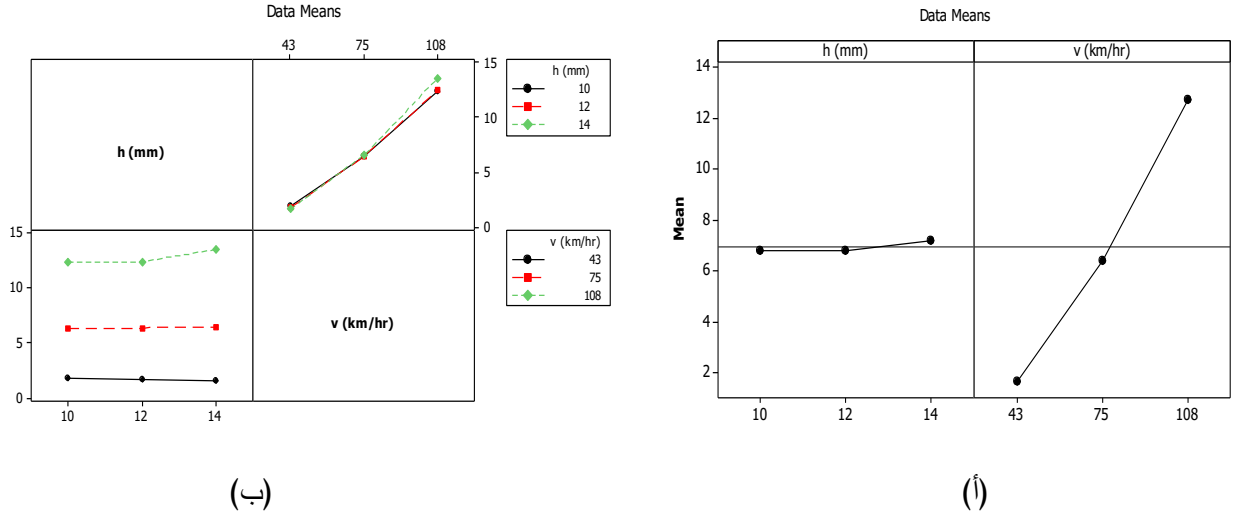
الشكل (٩) يمثل النتائج لفرق السائل في النقطة الخامسة ( \Delta H5 ), (أ) تأثير متوسط فرق السائل بتأثير السعة وارتفاع الموديل, (ب) شكل التفاعل في تغير مستوى القيم للعوامل المؤثرة على بعضها البعض.
