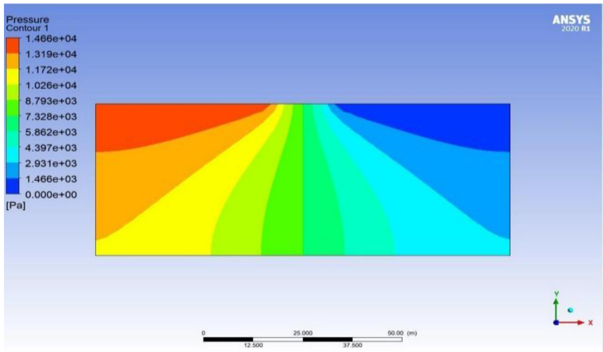
Figure 9. Equipotential lines
